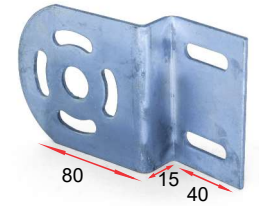
MANCAL ENTRE VÃO CHAPA 2,50 MM
