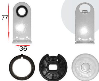
kit suporte para motor 38 / 53 mm
