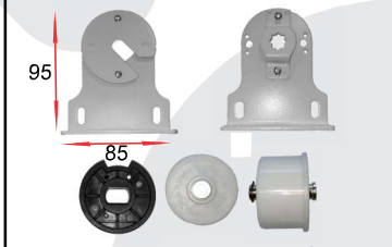
kit suporte para motor 53 / 70 mm
