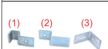
CADEIRINHAS DE FIXAÇÃO
