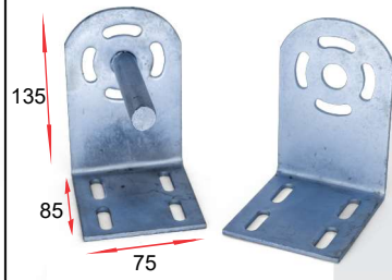
MANCAL TOLDO REFORÇADO CHAPA 3,10MM
