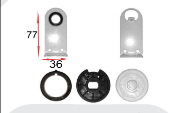
kit suporte para motor 38 / 53 mm
